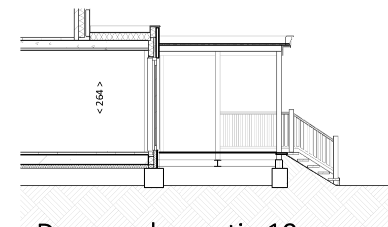
Doorsnede - optie 10 Schaal: 1 : 100
