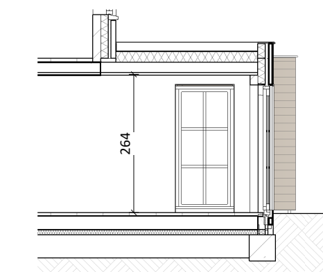
Doorsnede -optie 9 Schaal: 1 : 100
