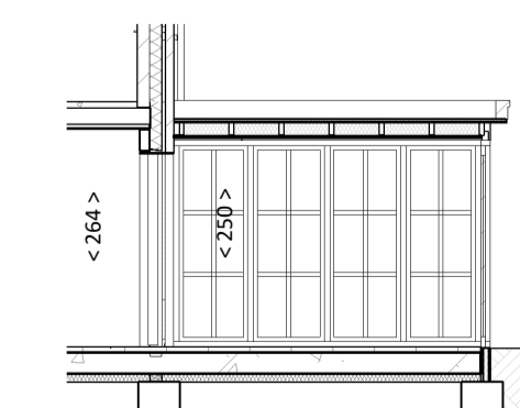
Doorsnede - optie 14
