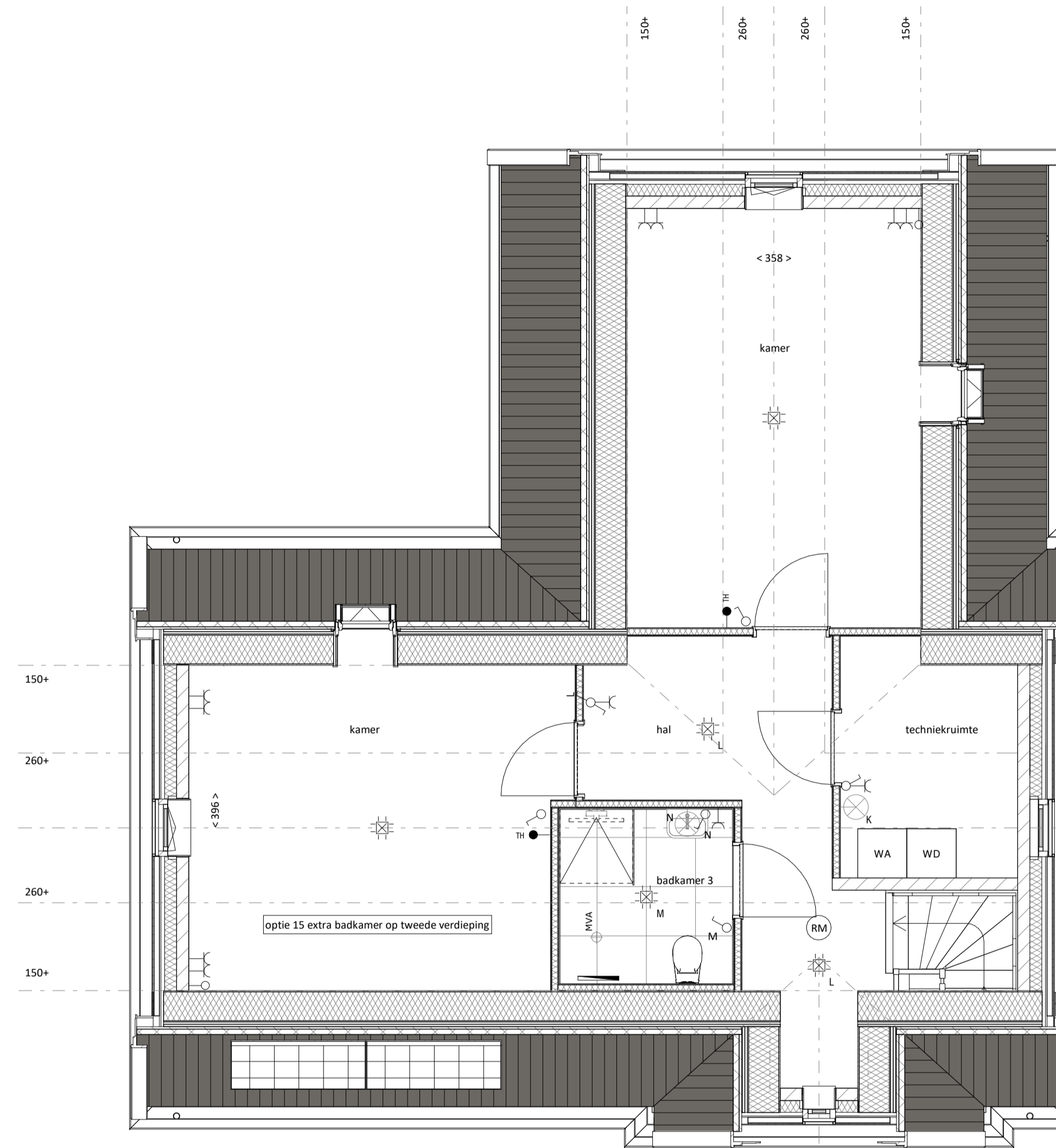
Tweede verdieping optie 15
